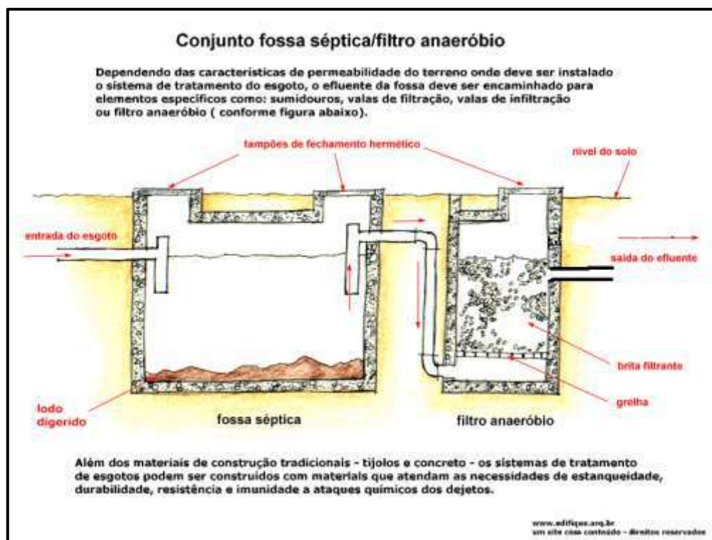
Figura 59: Fossa séptica de acordo com normal legais.
