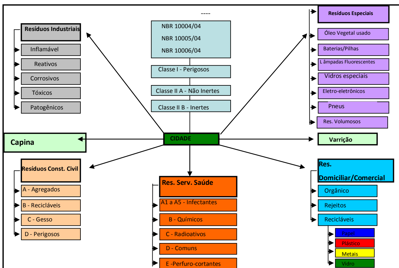
Figura 46: Fluxograma de um Sistema de Coleta/Transporte de Resíduos Sólidos Urbanos)
