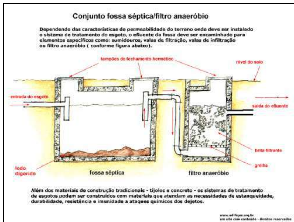
Figura 11: Fossa séptica de acordo com normal legais.
